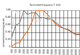
LI 12/4.0-1
