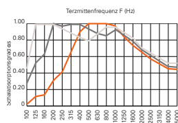
LI 13/3.0-1
