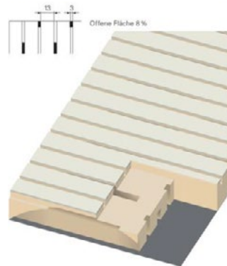
LI 13/3.0-1
