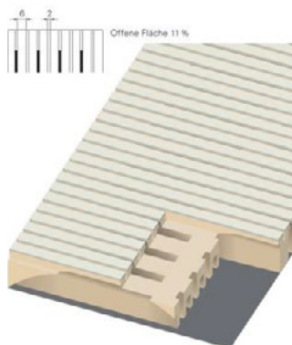
LI 6/2.0-1
