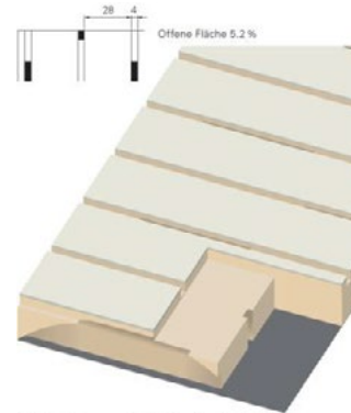
LI 28/4.0-1
