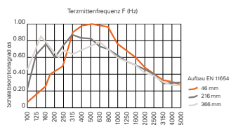
PE 16/16/3.0/5.0-1
