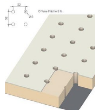
PE 32/32/8.0-1
