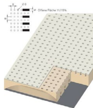
PE 8/8/3.0/5.0-1
