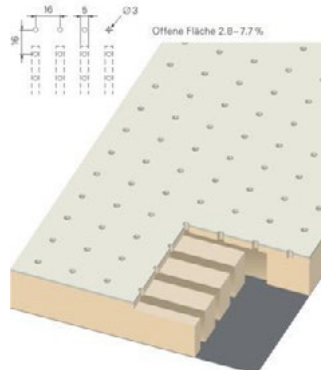
PE 16/16/3.0/5.0-1
